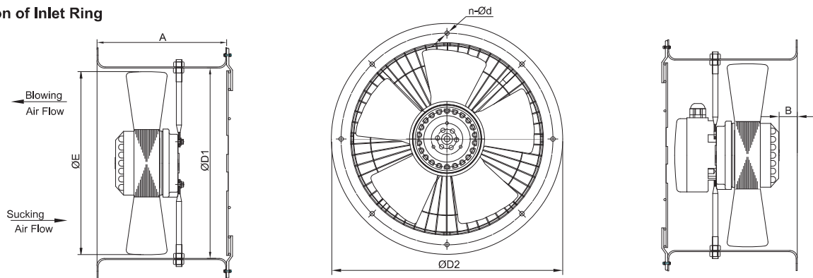
YWFXE/D-200S/B - YWFXE/D-450S/B
