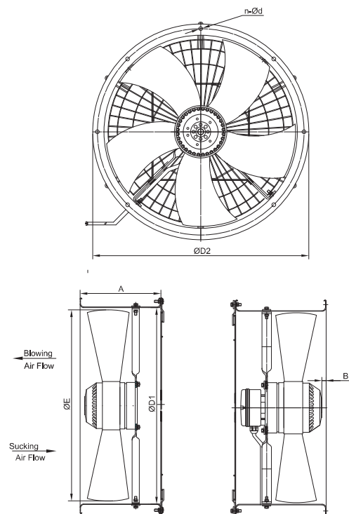
YWFXE/D-500S/B - YWFXE/D-630S/B
