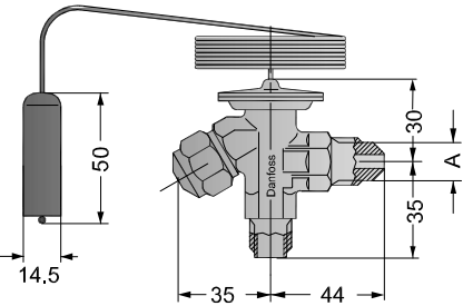
Figure: Flare × flare
